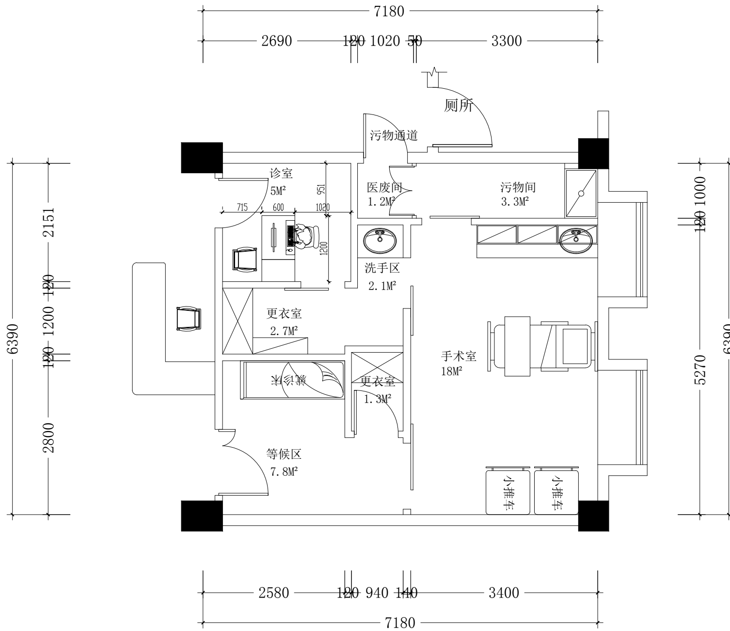
平面布置图(方案一)
